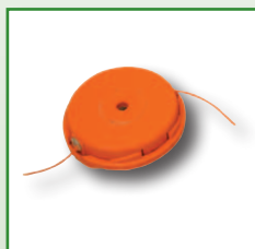
Coupe Ø 440 mm boîtier à fil Ø 2,5 mm système Tap & Go
